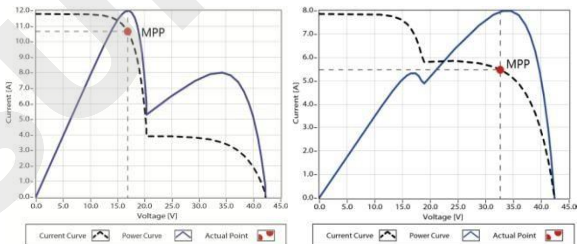
Рисунок 1-3 Кривая нескольких MPP
