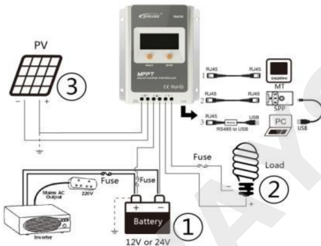
Рисунок 2-1 Монтаж
